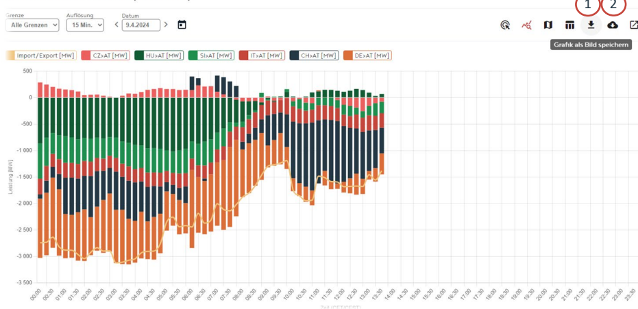
PHYSIKALISCHE LASTFLÜSSE (09.04.2024)
